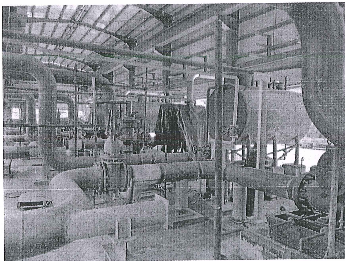
نمایی از تجهیزات واحد آب آتش نشانی (FWS)
