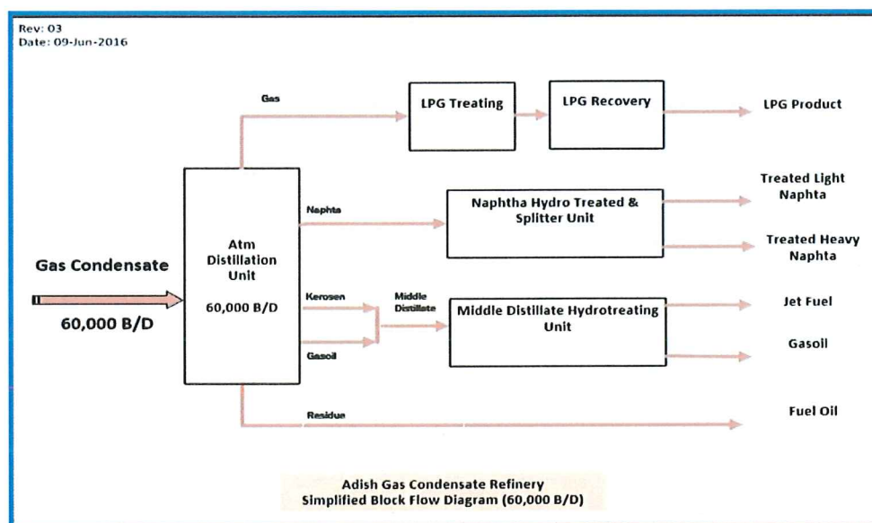
شکل ۵- نحوه ارتباط واحدهای مختلف پالایشگاه میعانات گازی آدیش جنوبی
