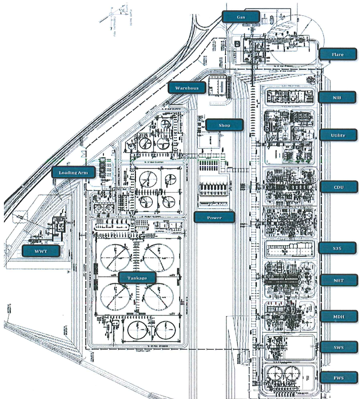
شکل ۴- لی اوت واحد
