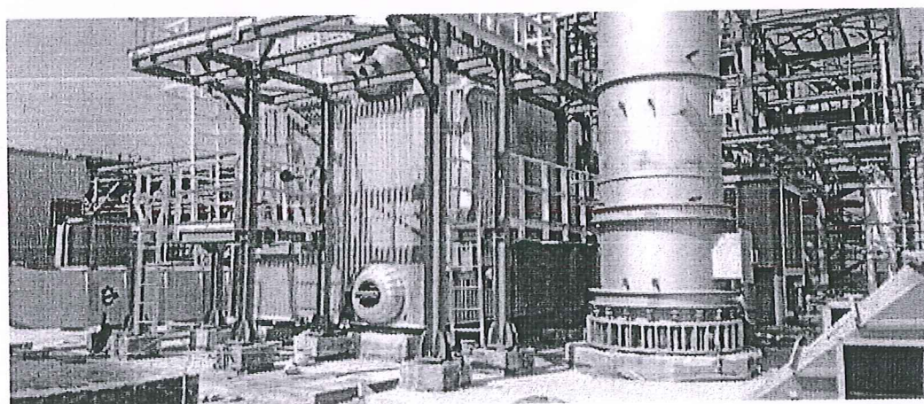
نمایی از وضعیت واحد یوتیلیتی (UTL)
