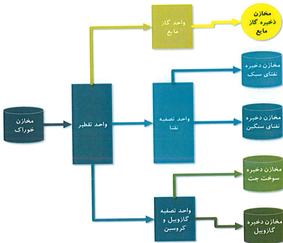
شکل ۷- نمای فرآیندهای پالایشگاه
