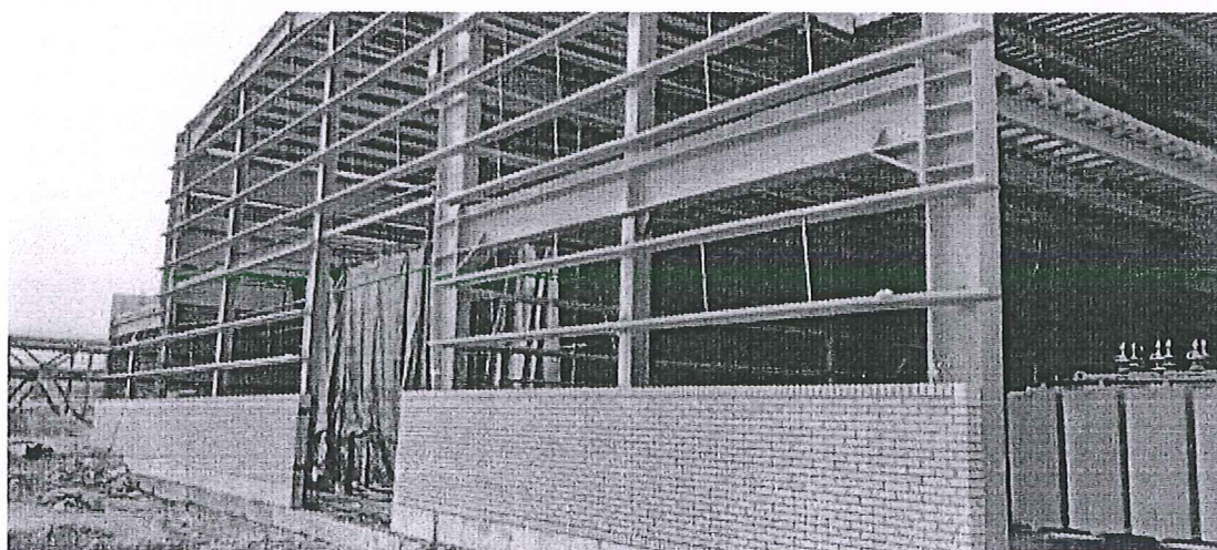
نمایی از وضعیت واحد نیروگاه (PGU)
