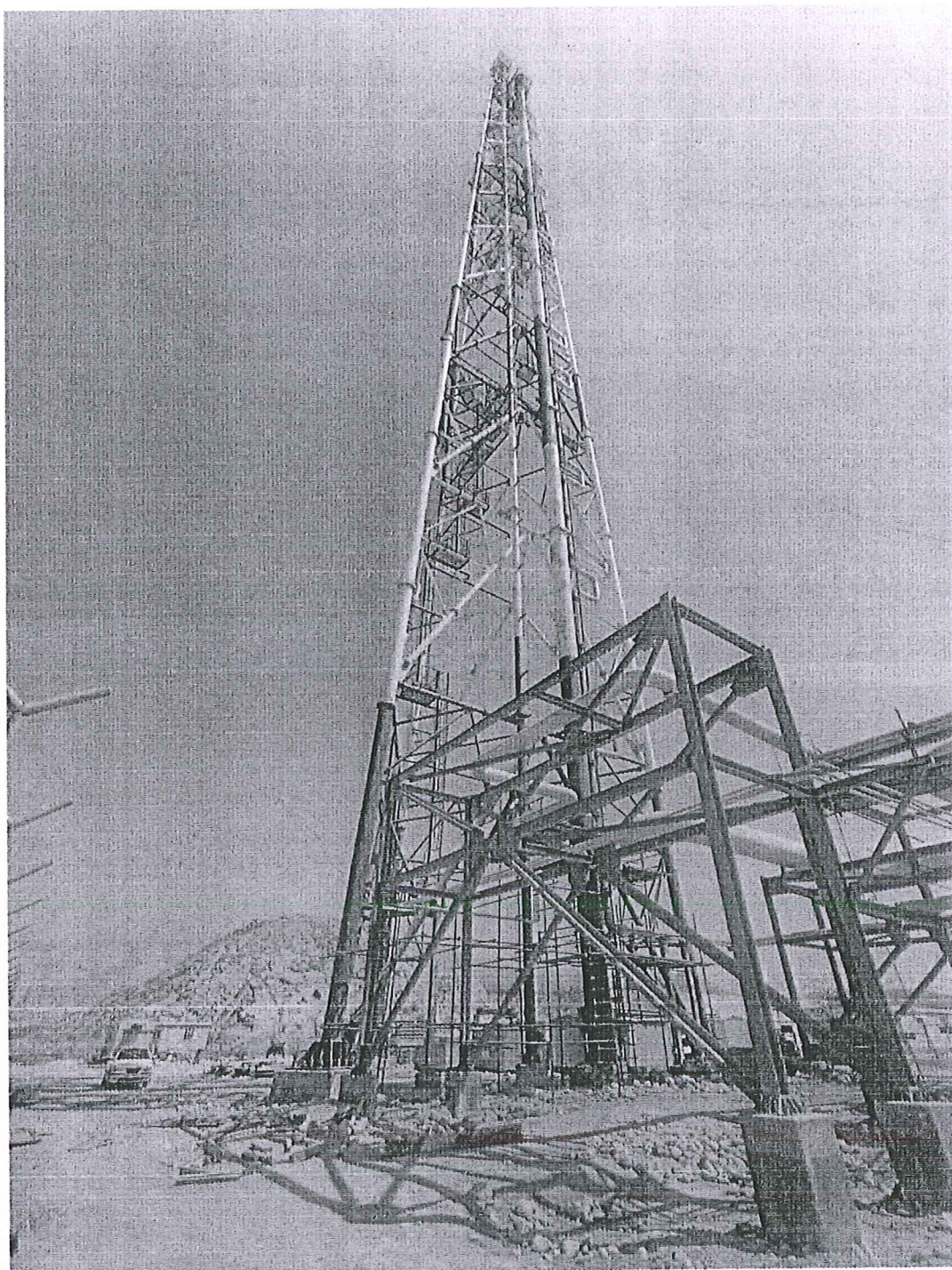
نمایی از وضعیت واحد فلر (FLS)
