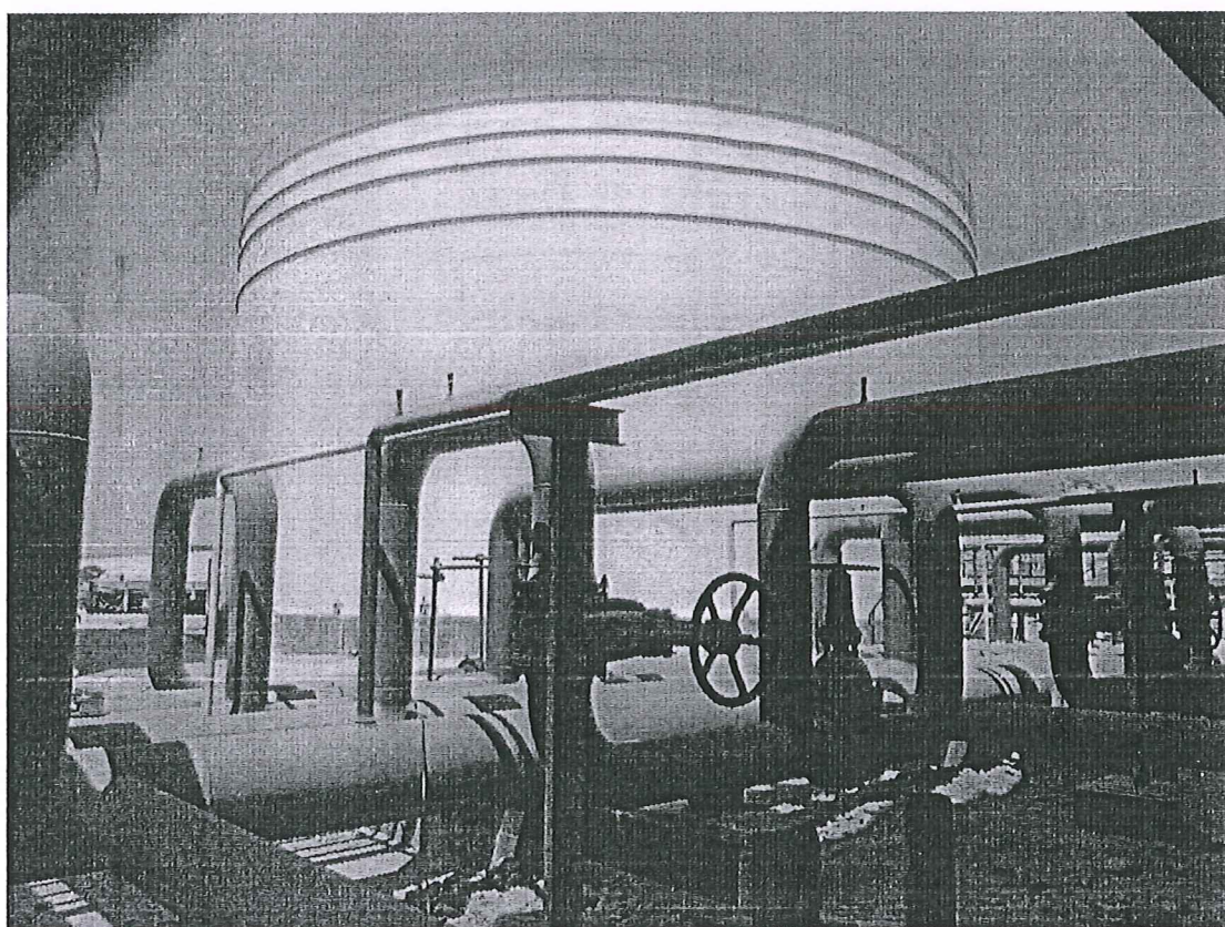
نمایی از مخازن و سیستم لوله کشی آب آتش نشانی
