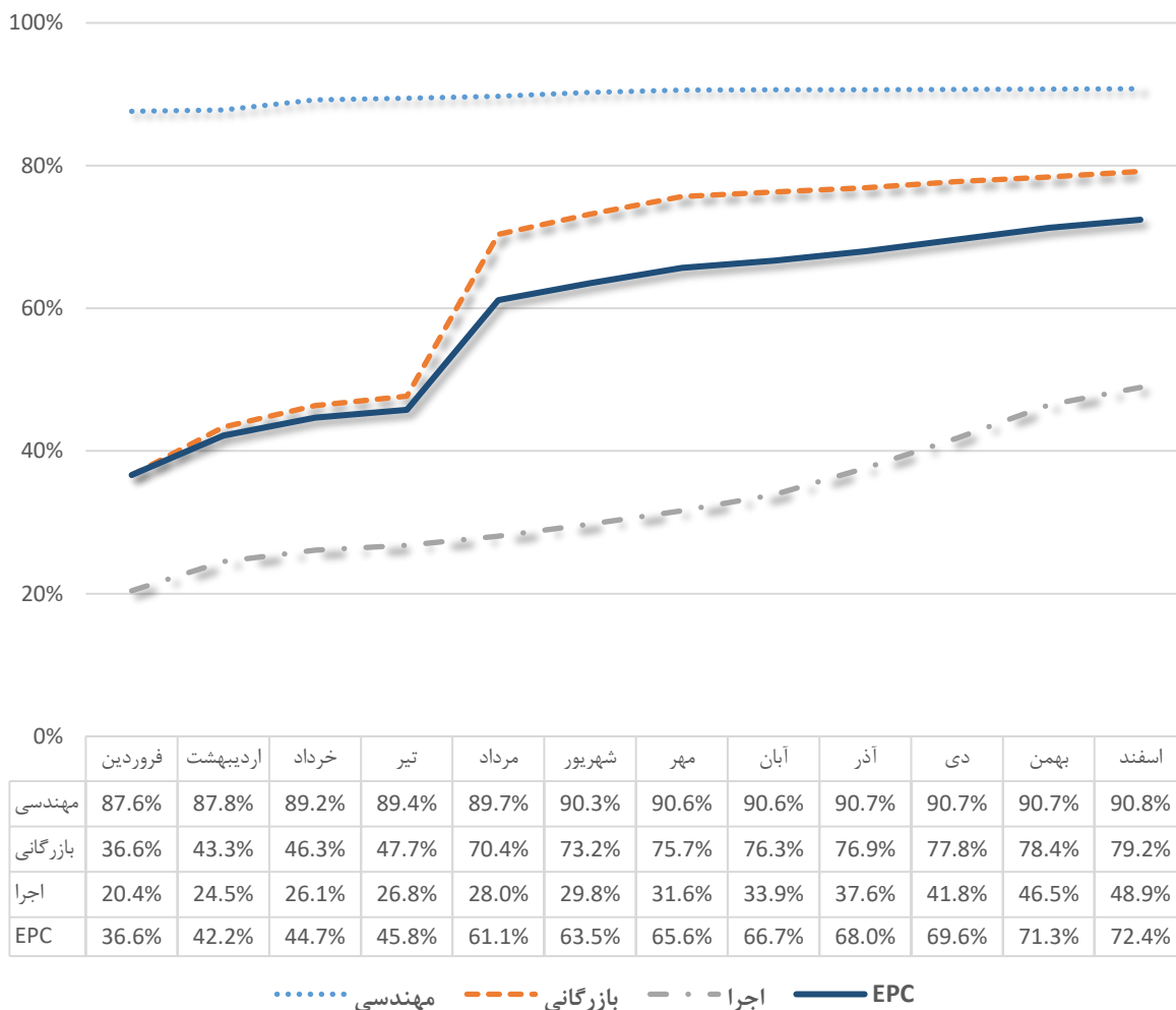
نمودار پیشرفت واقعی پروژه EPC - سال ۱۴۰۰
